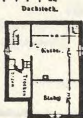
Wohnhaus für 2 kleine Familien (Witwenhäuser), System 6.
