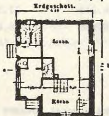
Wohnhaus für 2 kleine Familien (Witwenhäuser), System 6.
